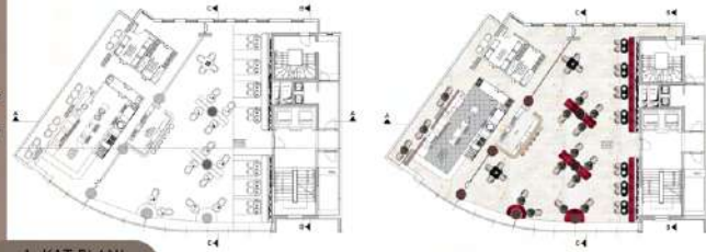
1. KAT PLANI 1/50
